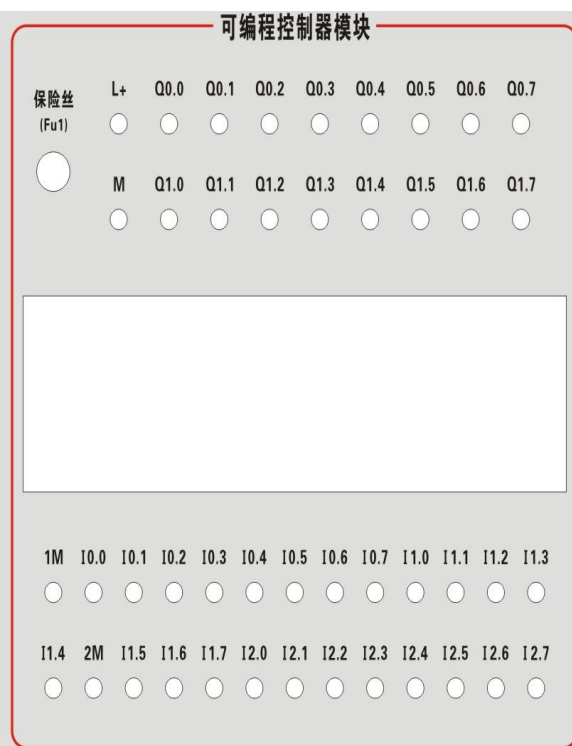
图 1-14-10 CPU226CN 可编程控制器模块
