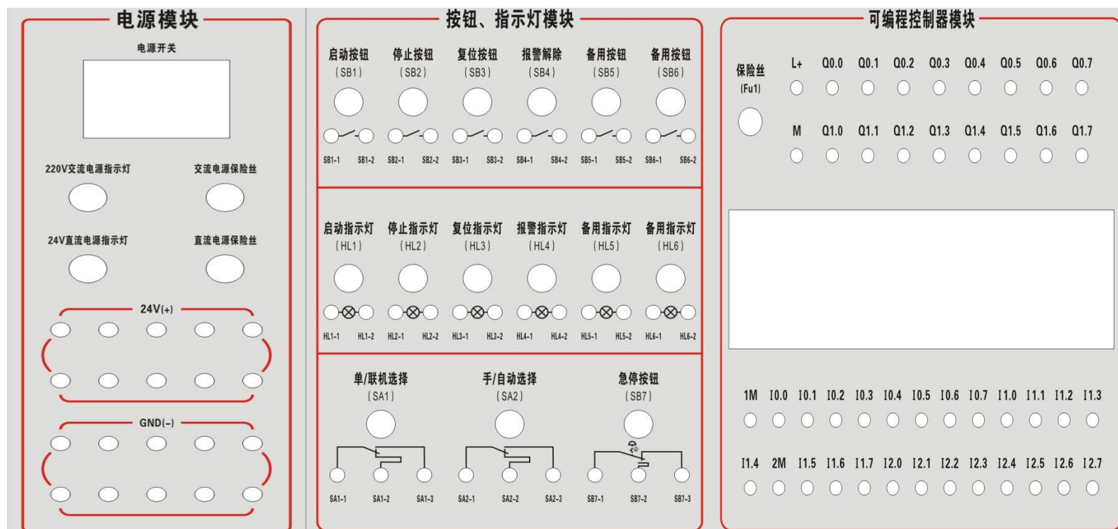
图 1-14-8 电源模块
