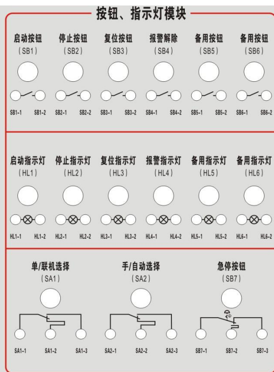
图 1-14-9 按钮、指示灯模块
