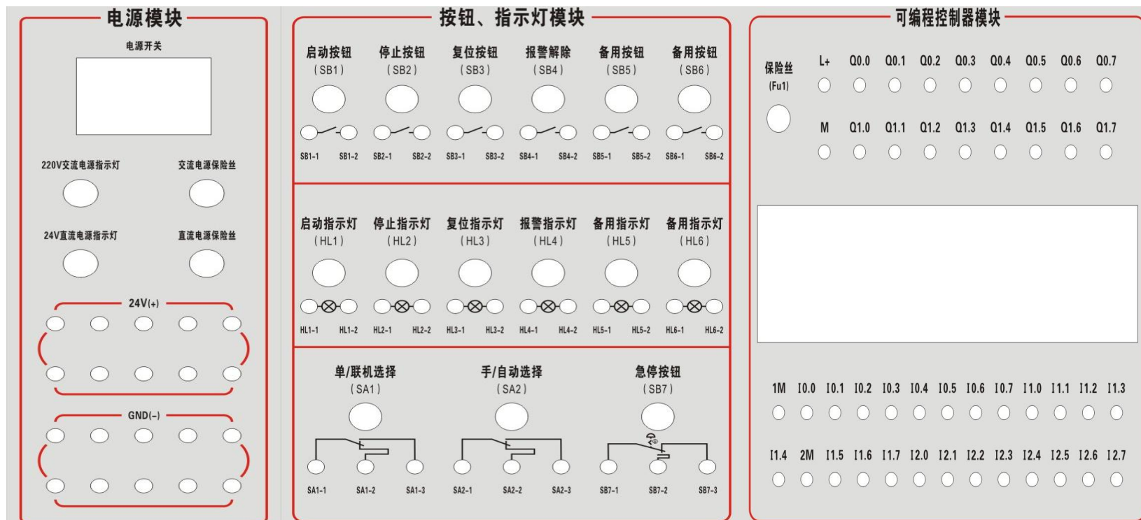
图 1-12-7 电源模块
