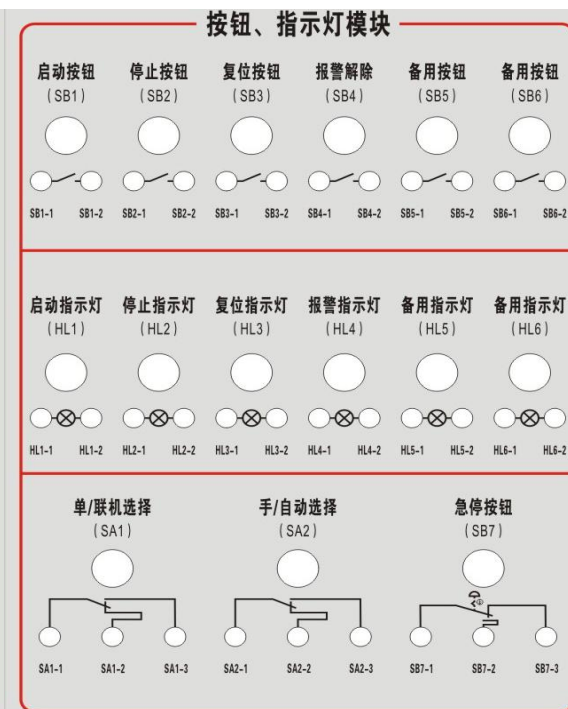
图 1-9-8 按钮、指示灯模块
