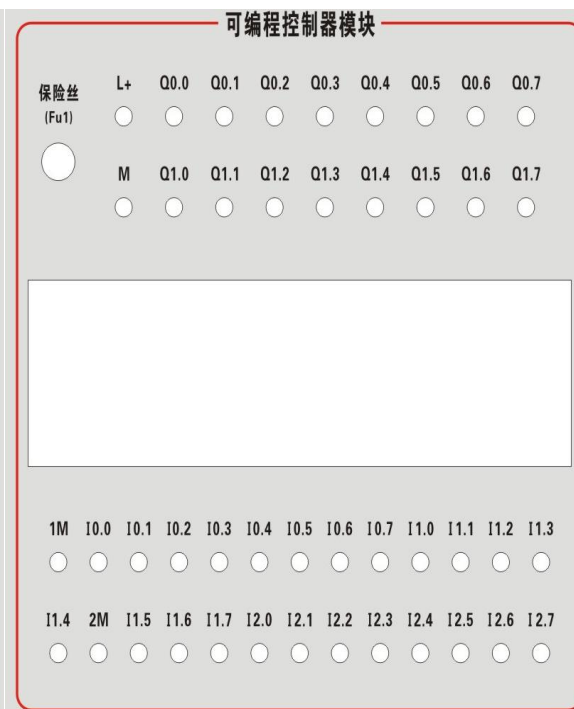
图 1-9-9 CPU226CN 可编程控制器模块
